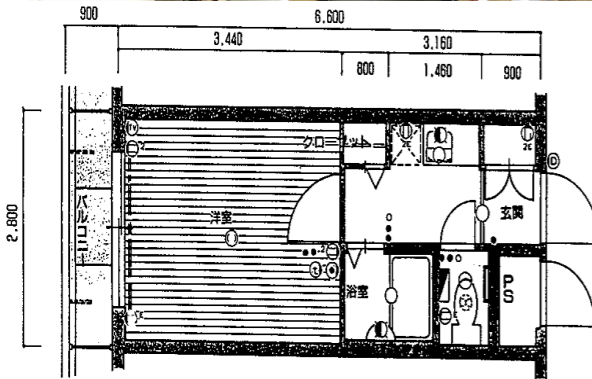
(122,132号室) Aタイプ ●専有面積/18.48㎡ ●バルコニー面積/2.52㎡ ※現況優先
