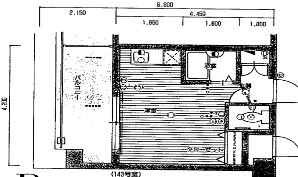
(143号室) Bタイプ ●専有面積/18.69㎡ ●バルコニー面積/6.30㎡
